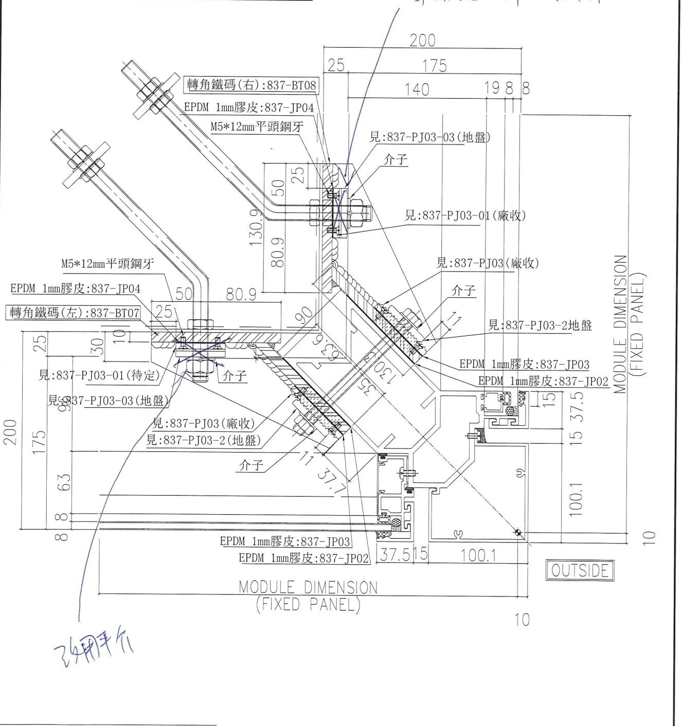
轉角鐵碼組合左右各一個鐵碼
