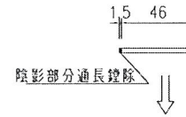
模號: ME0002318 名稱: 47.5X3鋁巴 合金狀態: 6063-T5 重量: 0.386KG/M V.F.: 53.5 mm
