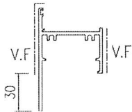
模號: X846180 名稱: 視底橫 合金狀態: 6063-T5 重量: 1.182KG/M V.F.: 91 mm
