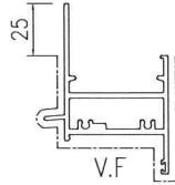
模號: X846150 名稱: 生頂橫(空腔) 合金狀態: 6063-T5 重量: 1.617KG/M V.F.: 193 mm
