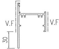
模號: X846180 名稱: 梗底橫 合金狀態: 6063-T5 重量: 1.182KG/M V.F.: 91 mm
