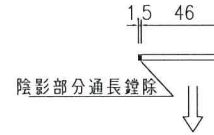
模號: ME0002318 名稱: 47.5X3mm 鋁巴 合金狀態: 6063-T5 重量: 0.386KG/M V.F.: 53.5 mm
