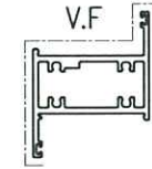
模號: X846100 名稱: 上生下梗中橫 合金狀態: 6063-T5 重量: 1.443KG/M V.F.: 178 mm
