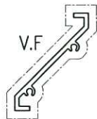
模號: X843331 名稱: 百葉片 合金狀態: 6063-T5 重量: 0.896KG/M V.F.: 238.5mm
