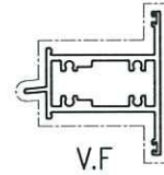
模號: X846080 ✓ 名稱: 上生下生中橫 合金狀態: 6063-T5 重量: 1.542KG/M V.F.: 276 mm
