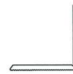
模號: X846100 名稱: 上生下梗中橫 合金狀態: 6063-T5 重量: 1.443KG/M V.F.: 178 mm
