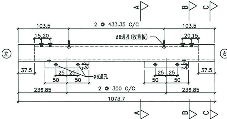
“D” 视图
