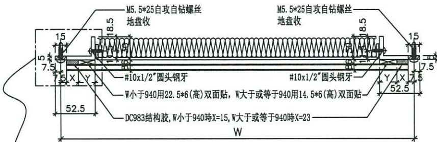
角码示意图
