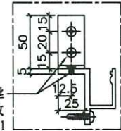
角码示意图
