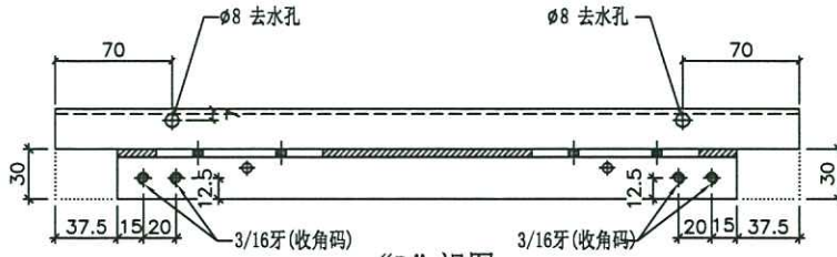
“D” 视图
