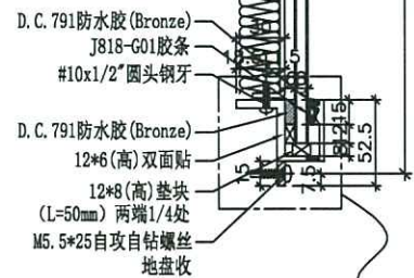
角码示意图
