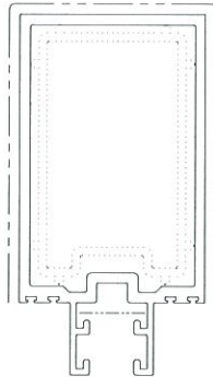
模號: X85545 名稱: 雙梗企 合金狀態: 6063-T6 重量: 7.276 KG/M V.F.: 423.14mm
