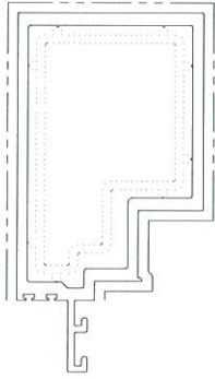
模號: X85546 名稱: 生梗企 合金狀態: 6063-T6 重量: 6.936 KG/M V.F.: 425.36mm
