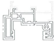
模號: X85581 名稱: SD框頂橫 合金狀態: 6063-T6 重量: 2.195 KG/M V.F.: 325 mm
