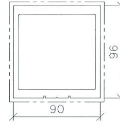
模號: X85548 名稱: SD中企 (外凹) 合金狀態: 6063-T6 重量: 6.48 KG/M V.F.: 379.9 mm
