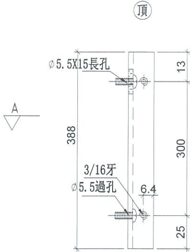
鋁角圖號:LJ-C04a
