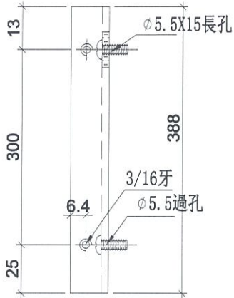
鋁角圖號:LJ-C04Ra
