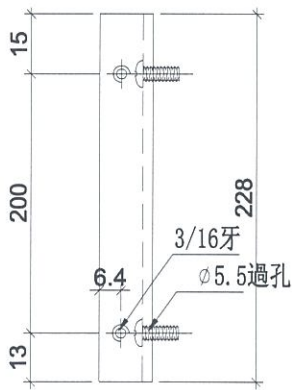
鋁角圖號:LJ-C04Rb
