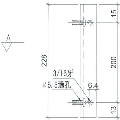
鋁角圖號:LJ-C04b
