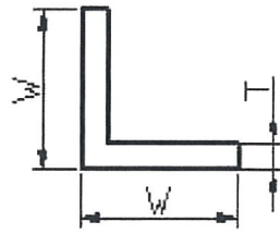
等边角
