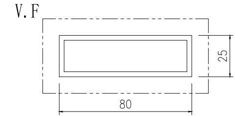
模號: ME0000566 名稱: 80x25x3mm厚鋁通 合金狀態: 6063-T5 重量: 1.604 KG/M V.F.: 210 mm
