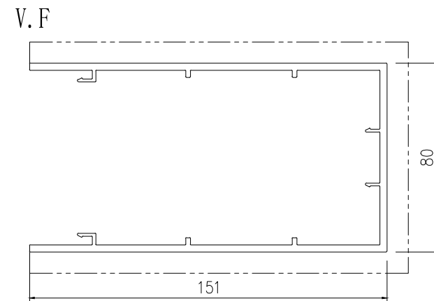
模號: X85633 名稱: 企向裝飾型材 合金狀態: 6063-T6 重量: 3.243 KG/M V.F.: 382.08 mm
