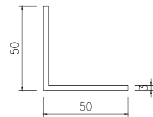
模號: ME0001961 名稱: 50x50x3mm厚鋁角 合金狀態: 6063-T6 & 6063-T4 重量: 0.788 KG/M V.F.: mm
