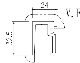
模號: X85615 名稱: 頂副框 合金狀態: 6063-T6 & 6063-T4 重量: 0.702 KG/M V.F.: 65.3 mm
