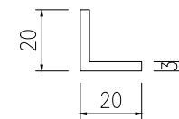
模號: PEOE10021 名稱: 20x20x3mm厚鋁角 合金狀態: 6063-T6 重量: 0.3 KG/M V.F.: mm
