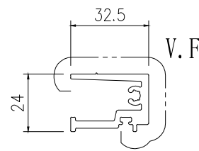
模號: X85612 名稱: 企副框 合金狀態: 6063-T6 重量: 0.765 KG/M V.F.: 65 mm
