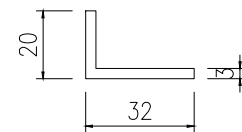
模號: ME0000018 名稱: 32x20x3mm厚鋁角 合金狀態: 6063-T6 & 6063-T4 重量: 0.397 KG/M V.F.: mm
