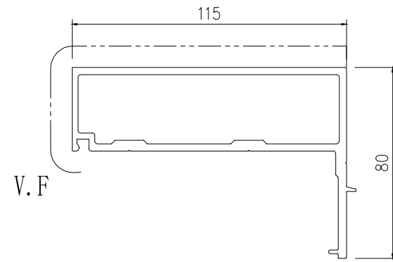
模號: X85611 名稱: 玻璃頂橫料 合金狀態: 6063-T6 重量: 2.923 KG/M V.F.: 175.76 mm
