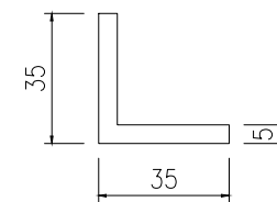
模號: LH0080096 名稱: 35x35x5mm厚鋁角 合金狀態: 6061-T6 重量: 0.881 KG/M V.F.: mm
