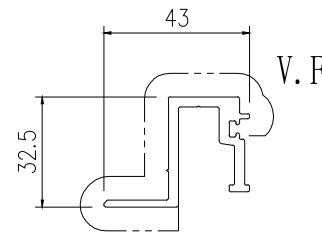
模號: X85613 名稱: 底副框 合金狀態: 6063-T6 重量: 0.807 KG/M V.F.: 0.103 mm
