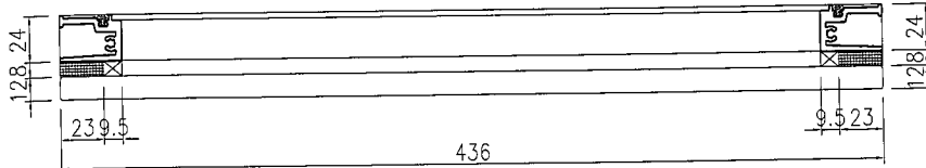
SECTION A-A
