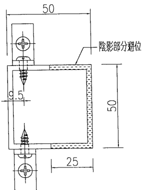
剖圖B-B
