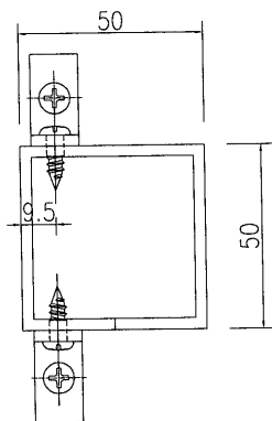
剖圖B-B
