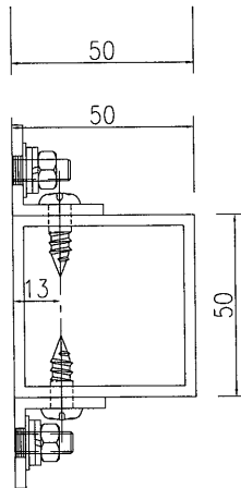
剖圖A-A
