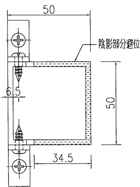
剖圖B-B
