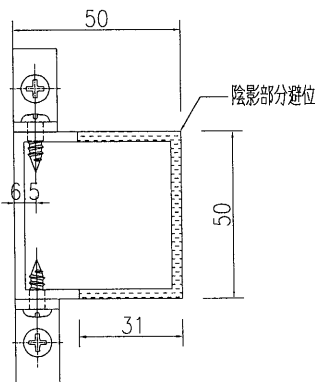
剖圖B-B
