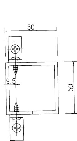
剖圖B-B
