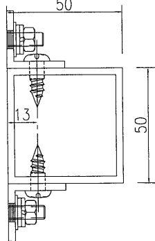
剖圖A-A
