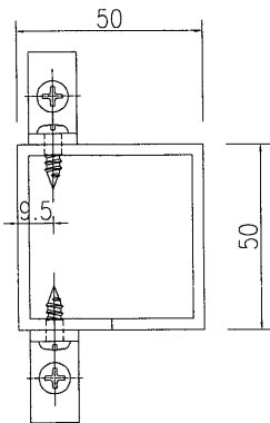
剖圖B-B
