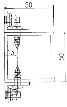
剖圖A-A
