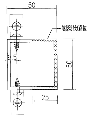
剖圖B-B
