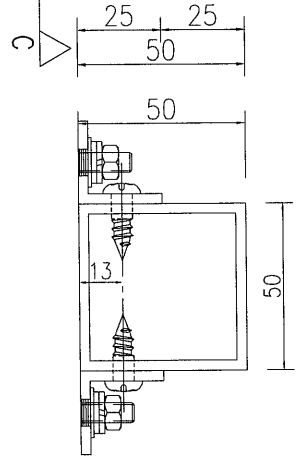
剖圖A-A
