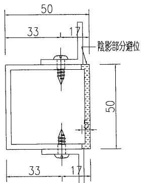
剖圖B-B
