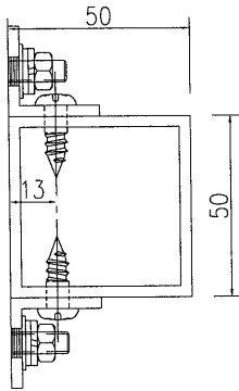
剖圖A-A
