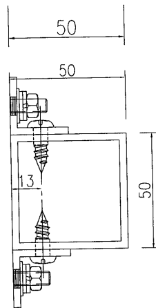
剖圖A-A
