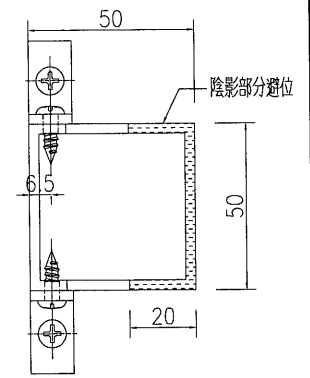
剖圖B-B
