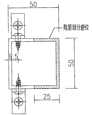
剖圖B-B
