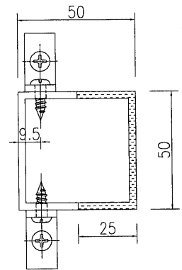
剖圖B-B
