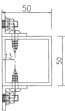
剖圖A-A
