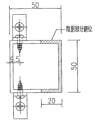
剖圖B-B
