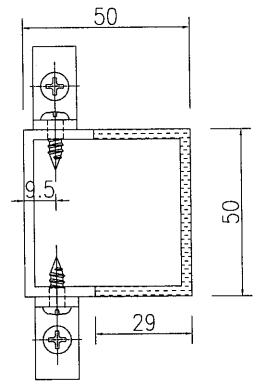
剖圖B-B
