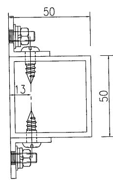
剖圖A-A
