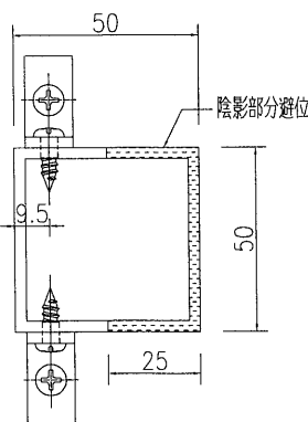
剖圖B-B
