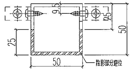
剖面B-B
