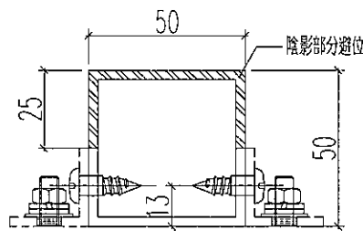
剖面A-A
