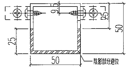
剖圖B-B
