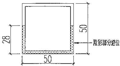
剖圖B-B
