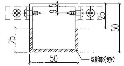
剖圖B-B
