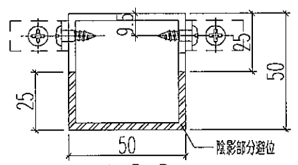
剖面B-B
