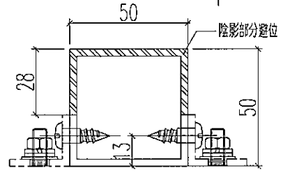
剖圖A-A
