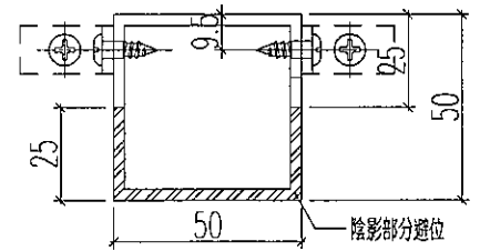
剖面B-B
