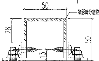
剖圖A-A
