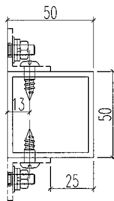
剖圖A-A
