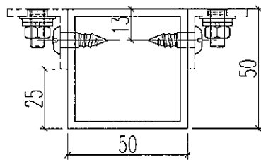
剖圖A-A
