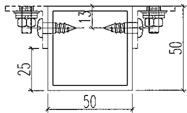
剖圖A-A
