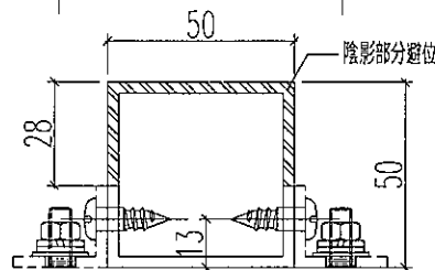
剖圖A-A
