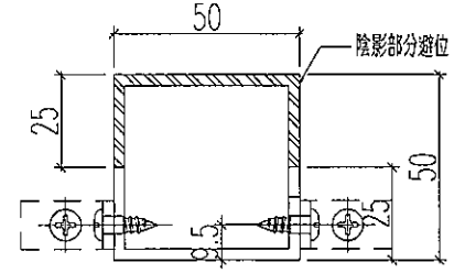
剖圖B-B
