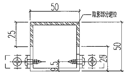
剖圖B-B
