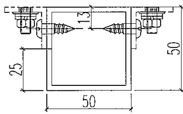
剖面A-A
