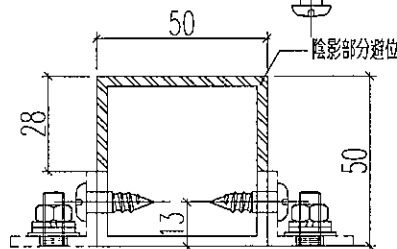
剖圖A-A
