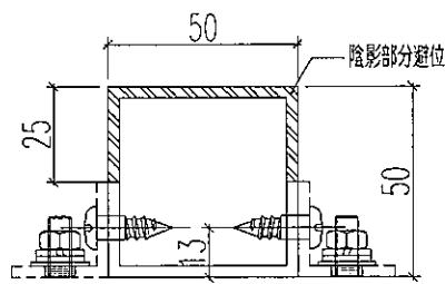
剖圖A-A
