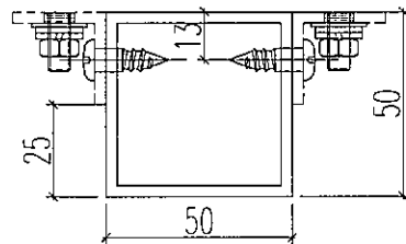
剖面A-A
