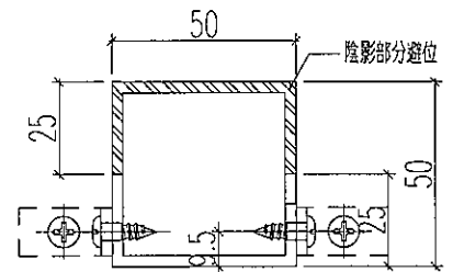
剖圖B-B
