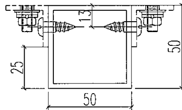
剖圖A-A
