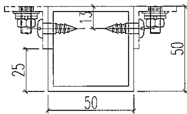
剖面A-A
