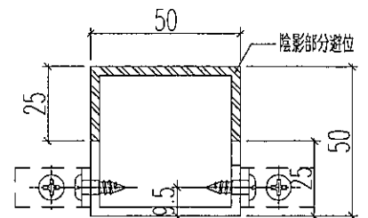
剖圖B-B
