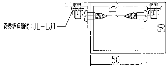
剖圖A-A
