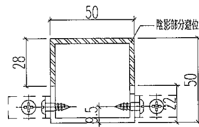
剖圖B-B
