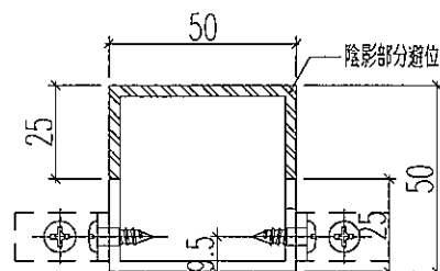
剖圖B-B
