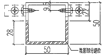
剖圖B-B
