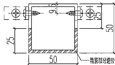
剖圖B-B
