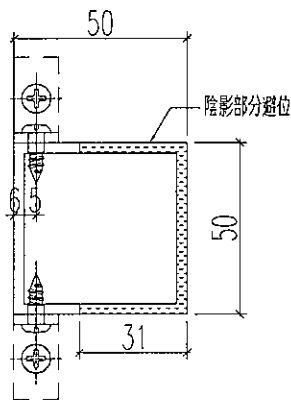
剖圖B-B
