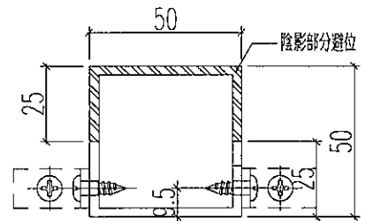
剖圖B-B
