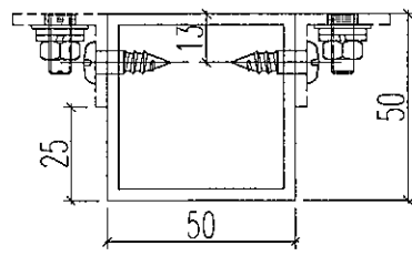
剖圖A-A
