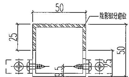
剖圖B-B
