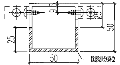
剖面B-B
