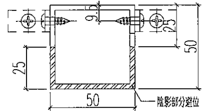
剖面B-B
