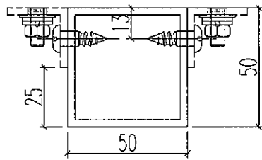
剖圖A-A
