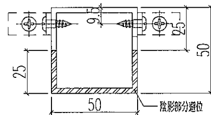
剖圖B-B
