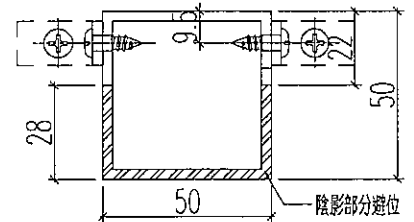
剖圖B-B
