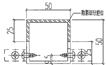
剖面B-B
