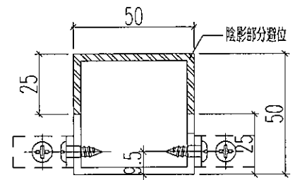
剖圖B-B
