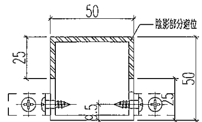
剖圖B-B
