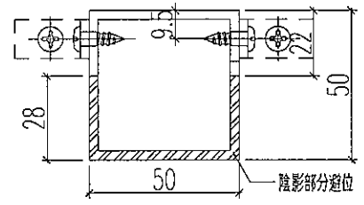
剖圖B-B
