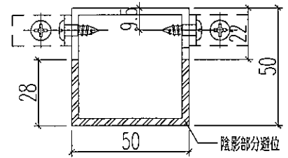
剖圖B-B
