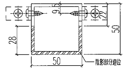
剖圖B-B
