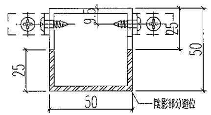
剖面B-B
