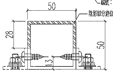
剖圖A-A
