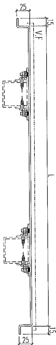
剖面圖 B-B
