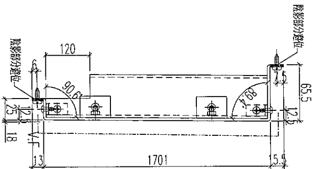
剖面A-A
