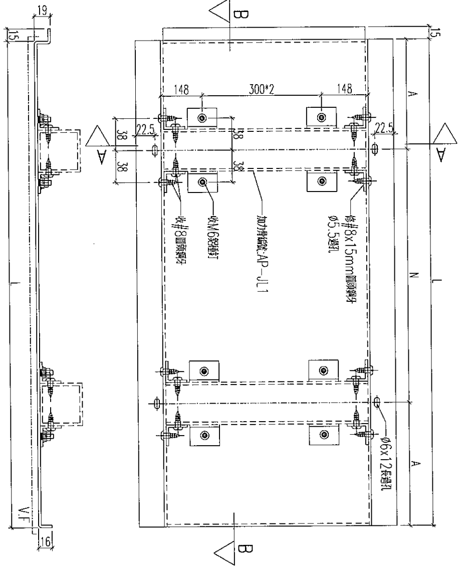
圖B-B
