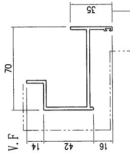
模號: X85617 名稱: 百葉頂框 合金狀態: 6063-T5 & 6063-T4 重量: 1.172 KG/M V.F.: 166.52 mm
