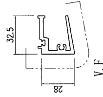
模號: X85659 名稱: 企副框 合金狀態: 6063-T6 重量: 0.822 KG/M V.F.: 69.8 mm
