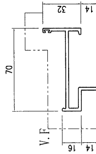
模號: X85616 名稱: 百葉底框 合金狀態: 6063-T5 & 6063-T4 重量: 0.961 KG/M V.F.: 135.52 mm
