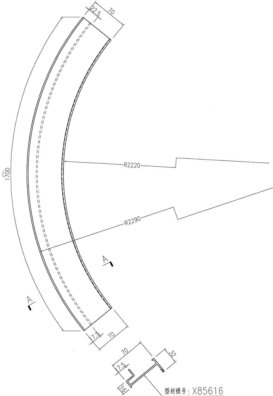
SECTION A-A
