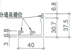
鏢料示意圖
