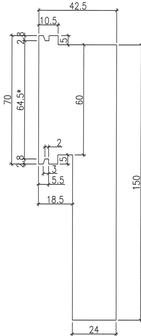
注：帶"*"號為重要尺寸
