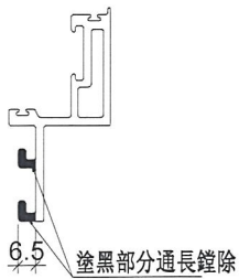
錠料示意圖
