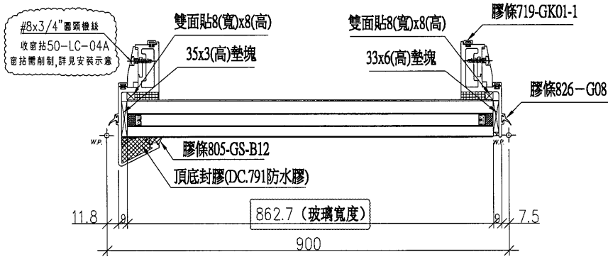
玻璃安裝示意圖
