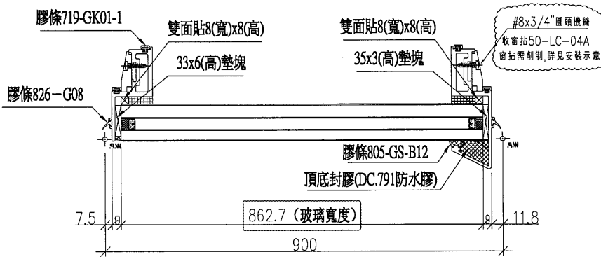
玻璃安裝示意圖
