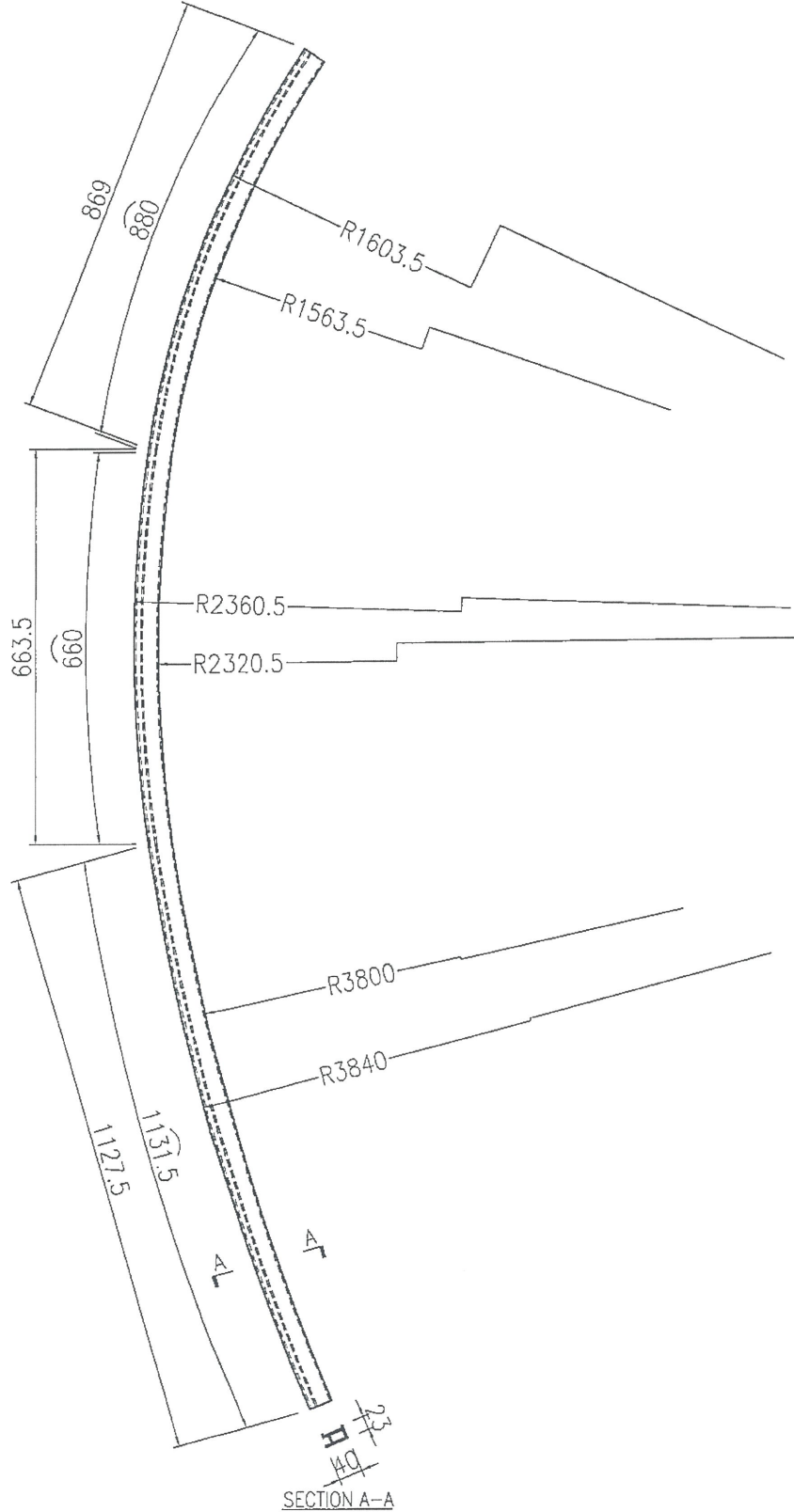
SECTION A-A
