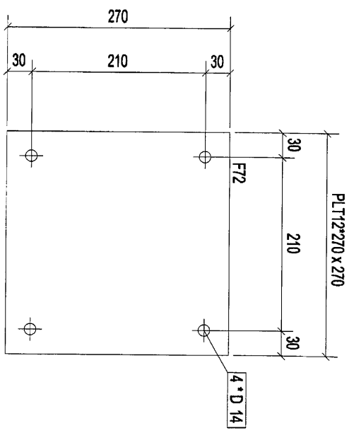
构件: ESJ-18
