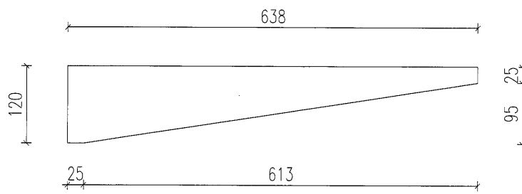
120x638x15mm THK. GMS PALTE 5.6kg/pc
