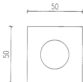
50x50x5mm THK. GMS PALTE 0.1kg/pc
