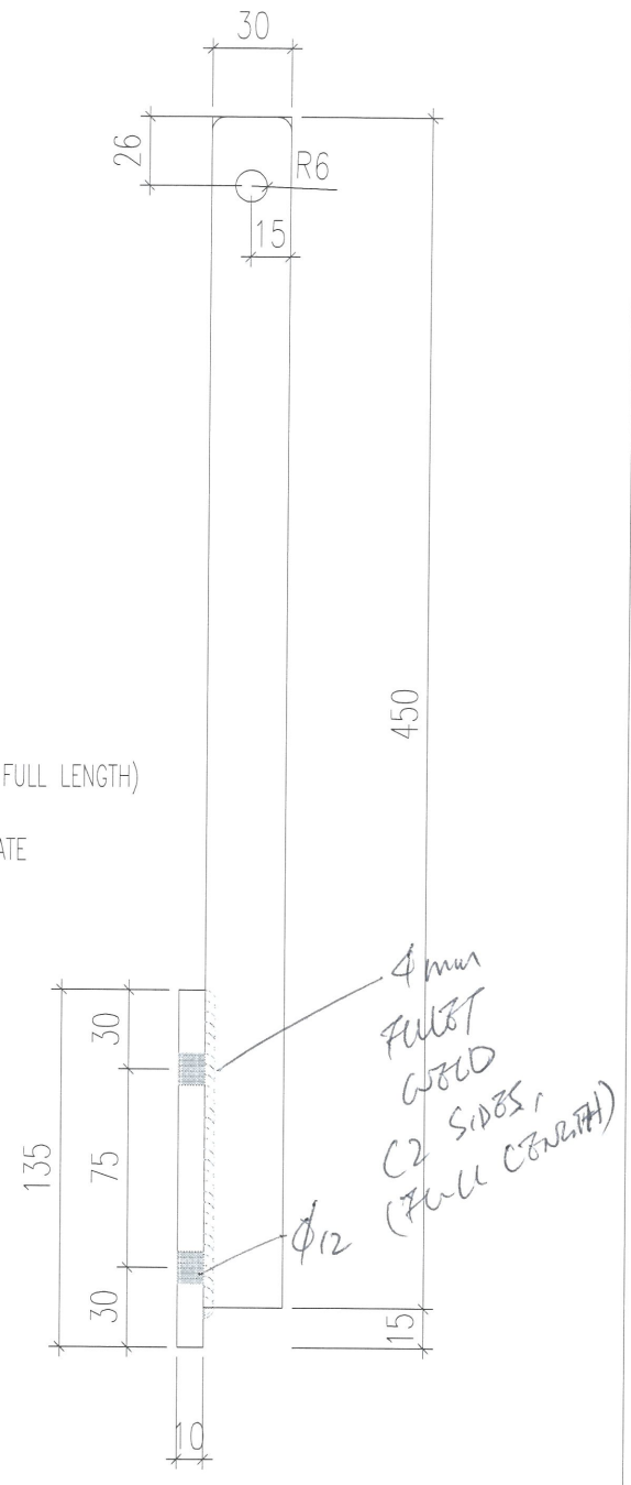
SECTION A-A
