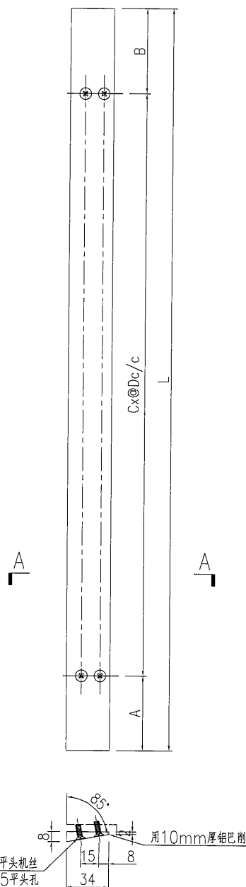
SECTION A-A
