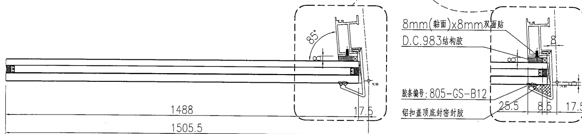
SECTION A-A
