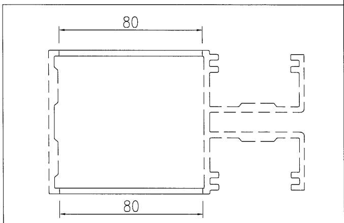
用型材X85368加工而成
