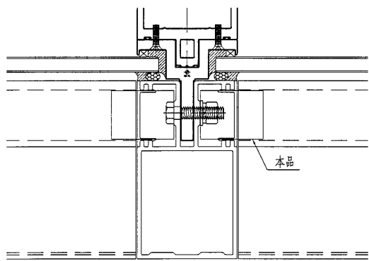
G/F十字装饰条交叉位用铝板挡胶铝板示意图
