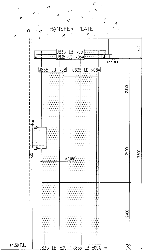
G 視圖
