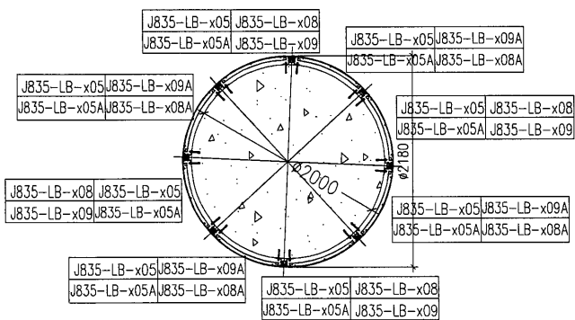
G 視圖
