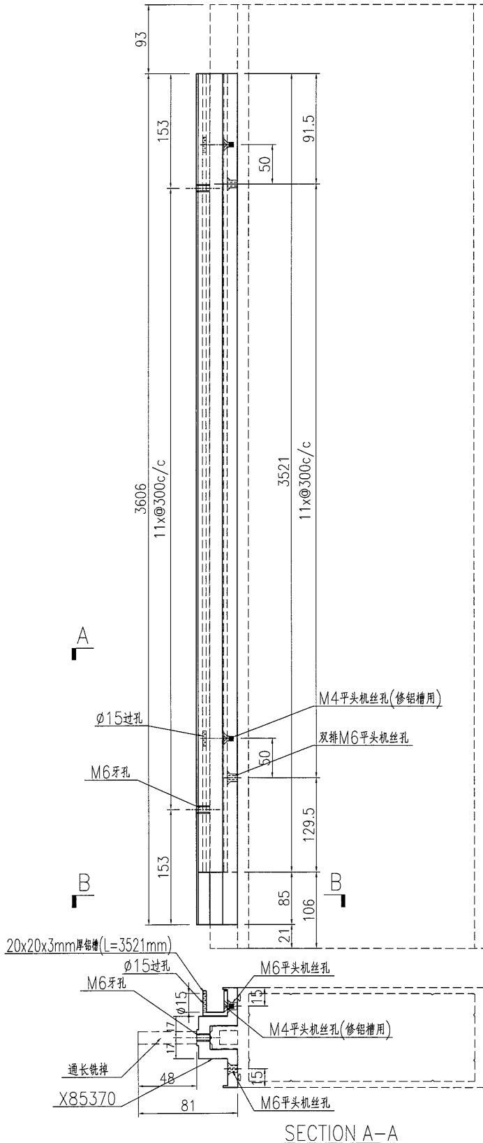
工厂组装示意图
