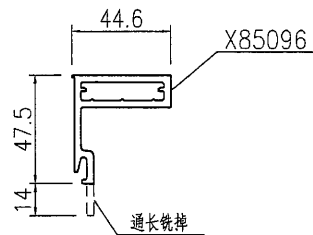
SECTION A-A 2:1
