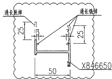
SECTION A-A 2:1
