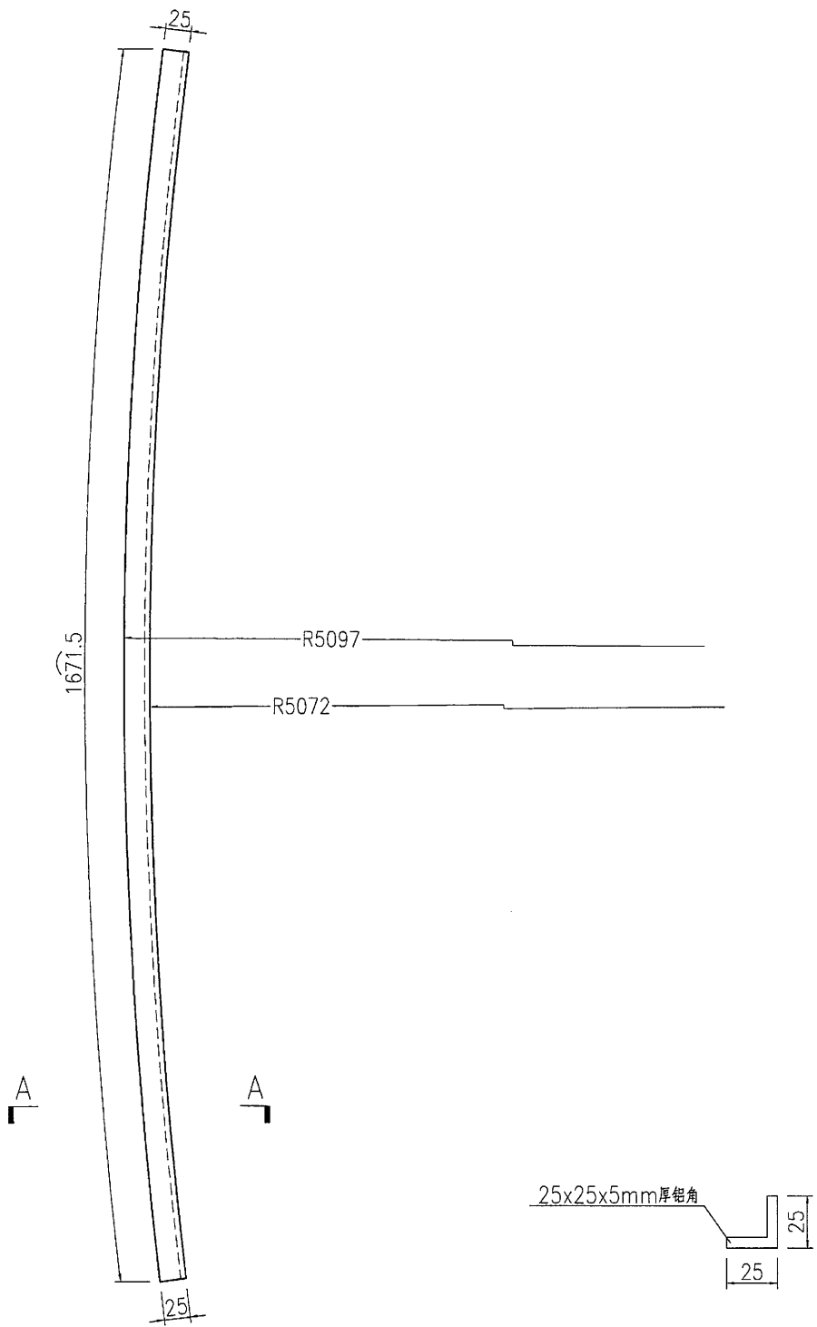
SECTION A-A 2:1
