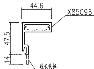
SECTION A-A 2:1
