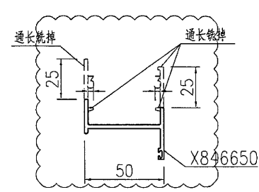
SECTION A-A 2:1
