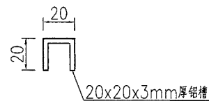
SECTION A-A 2:1
