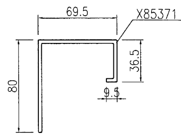
SECTION A-A 2:1
