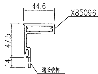
SECTION A-A 2:1
