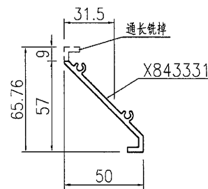
SECTION A-A 2:1
