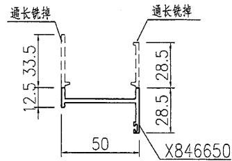
SECTION A-A 2:1
