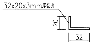
SECTION A-A 2:1
